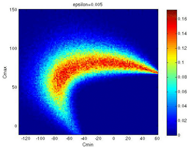
FIGURA 1. Fracción de matrices \rho_\epsilon^E entrelazadas (en escala de colores) encontradas en 1000 matrices \rho_1^E generadas aleatoriamente (como es descrito en la sub-sección 2.1) dentro de cada intervalo \langle C_{\min}, C_{\max} \rangle ; fueron considerados 130 valores tanto para C_{\min} como para C_{\max} , siendo el valor del parámetro usado igual a \epsilon = 5 \times 10^{-3} .
