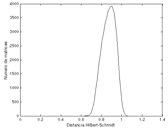
FIGURA 2. Histograma del número medio de matrices seudopuras extendidas y entrelazadas que tienen una distancia de Hilbert-Schmidt dada al “estado gato”, considerando \epsilon = 5 \times 10^{-4} . Se generaron (aleatoriamente) 500,000 matrices en cada ciclo de cálculos y se realizó un promedio sobre 10 ciclos.
